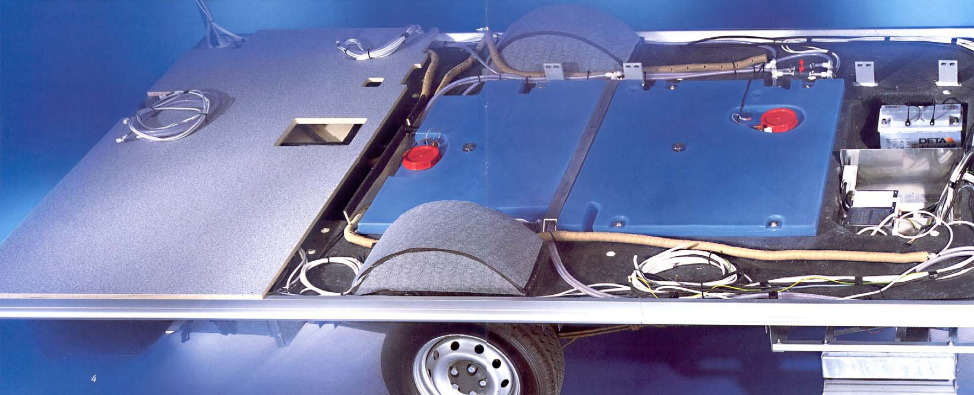
Im beheizten und isolierten Funktionsboden sind Wassertank, Abwassertank und Aufbau-Batterien versenkt integriert. Die Versorgungsleitungen verlaufen geschützt innerhalb der GFK-Formschale.
