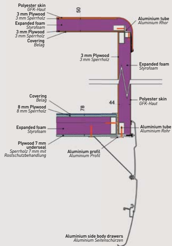
PLATINUM ON MERCEDES BASE SIMPLE FLOOR 5T3 PLATINUM AUF MERCEDES CHASSIS EINFACHBODEN 5T3
