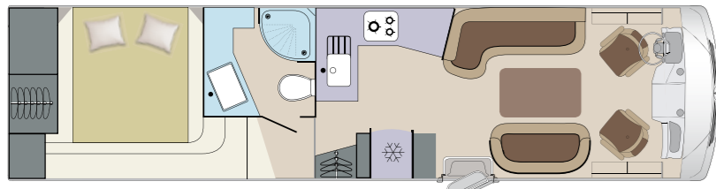
Featured vehicle with cream leather and India wood furniture Dargestelltes Fahrzeug mit Beige Leder und India Holzfarbe
