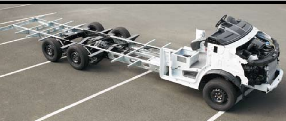
CHASSIS 6 WHEELS / FAHRGESTELL MIT 6 RÄDERN MB Sprinter 619 with rear wheel drive, double rear axles, air suspension and automatic gearbox (standard) on the models RX 10000, RX 11000 and RX 12000. MB Sprinter 619 mit Heckantrieb, hintere Doppelachsen, Luftfedern und Automatikgetriebe serienmäßig auf den Modellen RX 10000, RX 11000 und RX 12000.
