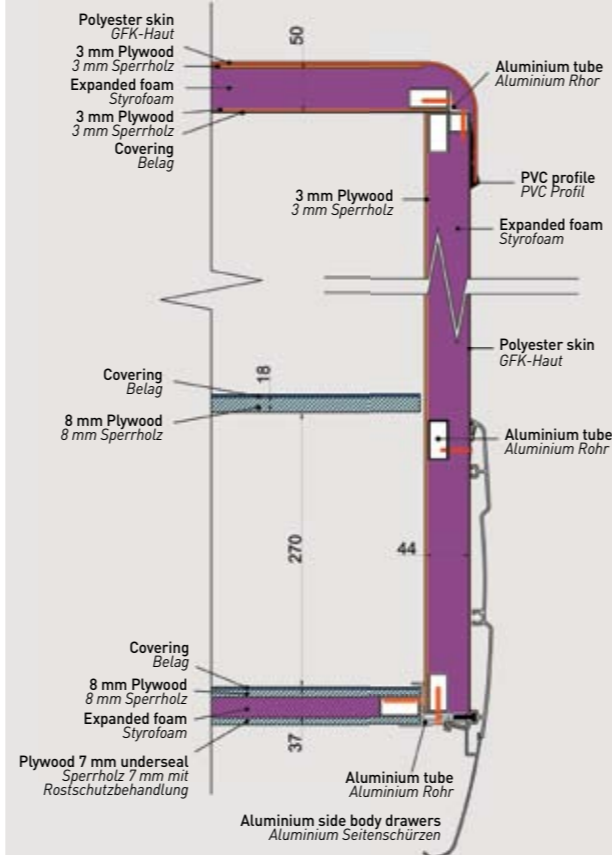
PLATINUM ON AL-KO BASE DOUBLE FLOOR 6T PLATINUM AUF AL-KO CHASSIS DOPPELBODEN 6T
