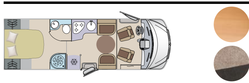
Featured vehicle with Savane upholstery and pear tree wood furniture Dargestelltes Fahrzeug mit Savane Stoff und Holzfarbe Birnbaum
