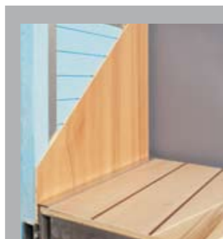
High quality coachwork with a sandwich-structure in Duralinox/Styrofoam of 45 mm guaranteeing rigidity to a maximal torsion. / Höchste Qualität für den Aufbau mit einer Sandwich-Struktur, die sich in Duralinox/Styrofoam bewährt hat. Die Seiten sind 45 mm stark und gewähren eine hohe Stabilität gegen eine maximale Torsion.
