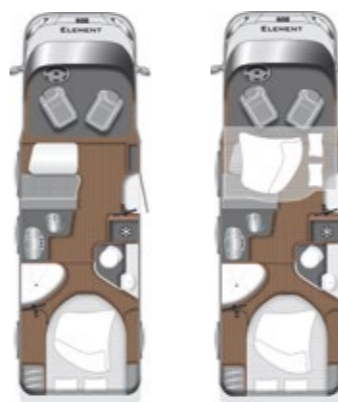
T 608 Longueur totale mm 6.980 Largeur totale mm 2.320 Nombre de couchages 2 (3/5)
