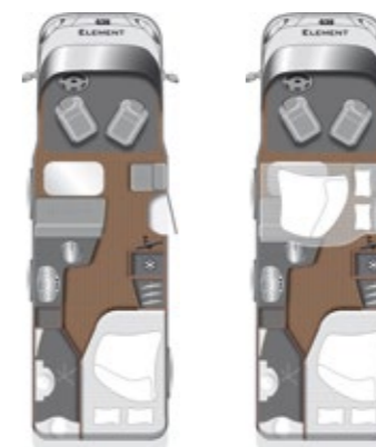
T 638 Longueur totale mm 6.980 Largeur totale mm 2.320 Nombre de couchages 2 (3/5)
