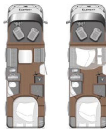
T 748 Longueur totale mm 7.410 Largeur totale mm 2.320 Nombre de couchages 2 (4)
