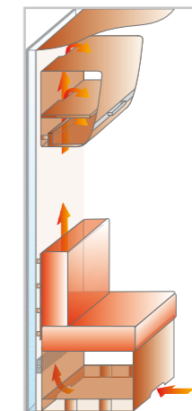
Durchdachtes Hinterlüftungskonzept (Serie)
