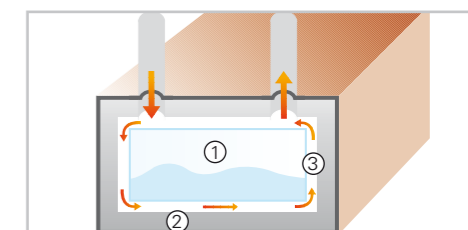
Isobox 1. Frisch-/Abwassertank 2. Isolierung 3. Warmluftzirkulation
