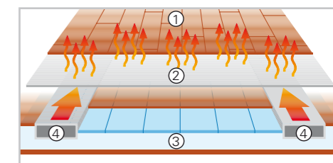
Fußbodentemperierung (Option) 1. Fußbodenbelag 2. Aluminiumwärmeleiter 3. Wärmedämmung 4. Heizungsrohr
