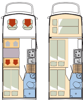
Ontario 635 LB/GB
