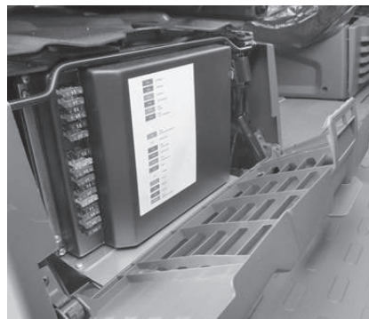
Occupation des fusibles
