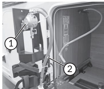
Régulateur de gaz
