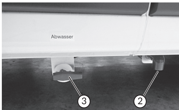
Écoulement des eaux usées (exemple Vantana)
