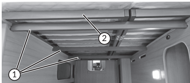
Positionnement de la barre transversale et du sommier à lattes Vantana
