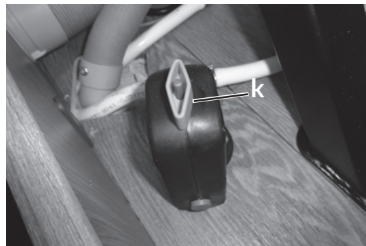
Soupape de sécurité pour chauffe-eau (FrostControl)
