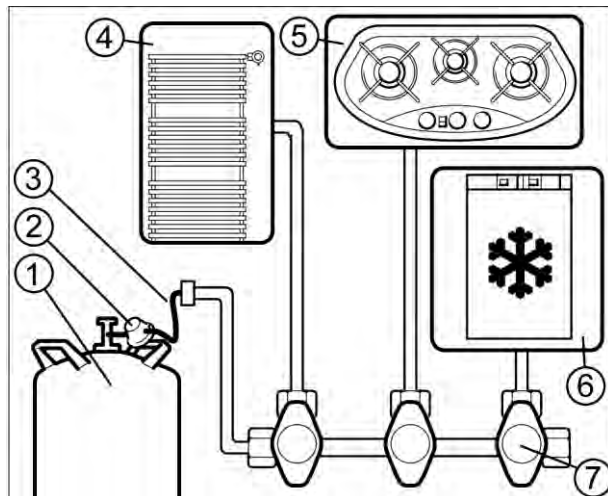
Gasanlage (schematisch)
