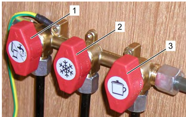
Schnellschlussventile
