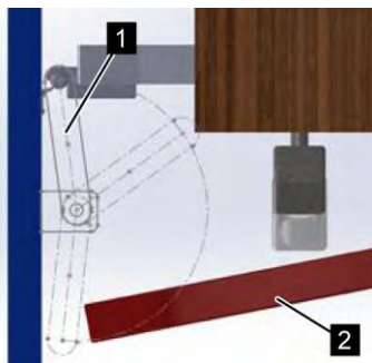
Drehgelenk Tischplatte
