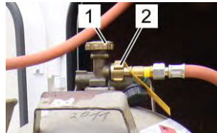
Anschluss Gasflasche
