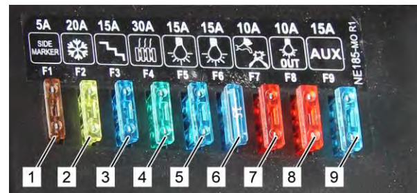
Verteilungsmodul NE185
