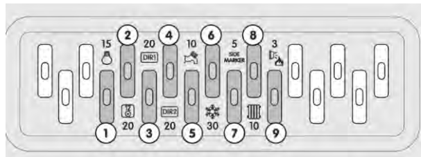
Verteilungsmodul RB450
