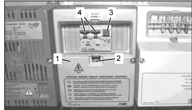
Sicherungsautomat mit FI-Schutz (Beispielabbildung)
