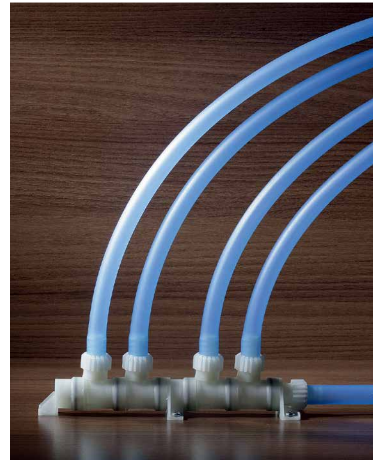
» Toutes les lignes de distribution en eau propre sont raccordées en un même point
