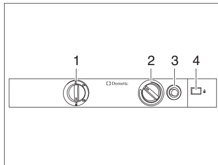
Fig. 243 Boutons de commande pour le réfrigérateur (Dometic Série 8)
