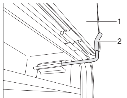
Fig. 53 Crochet de sécurité du portillon extérieur, position de blocage
