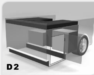
D2 Soute garage sous lit simple avec rallonges de châssis sur- baissé
