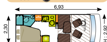
I 690 LP - I 691 LP AL-KO
