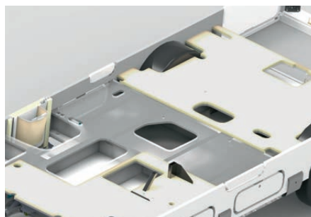
Le double plancher RAPIDO est solidaire du châssis abaissé AL-KO : son centre de gravité très bas assure une parfaite stabilité de conduite.
