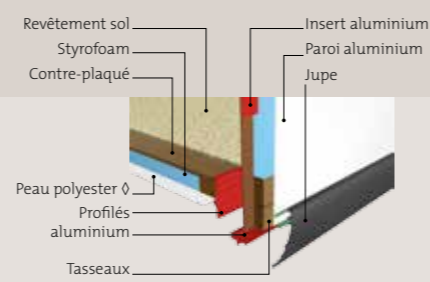
PROFILÉ SIMPLE PLANCHER
