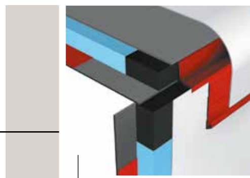
Jonction du toit et des parois latérales à l'aide de profilés aluminium
