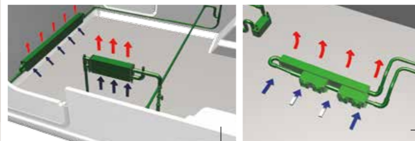
Régulateur thermique
