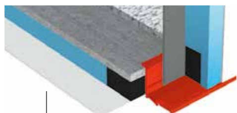
Structure plancher (cellule quasi autoportante) avec peau polyester** pour une meilleure isolation thermique et une protection renforcée contre l'humidité
