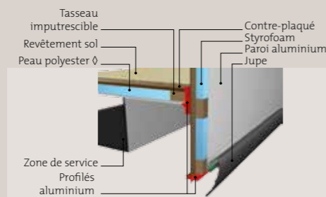
INTÉGRAL DOUBLE PLANCHER SERVICE 150 MM
