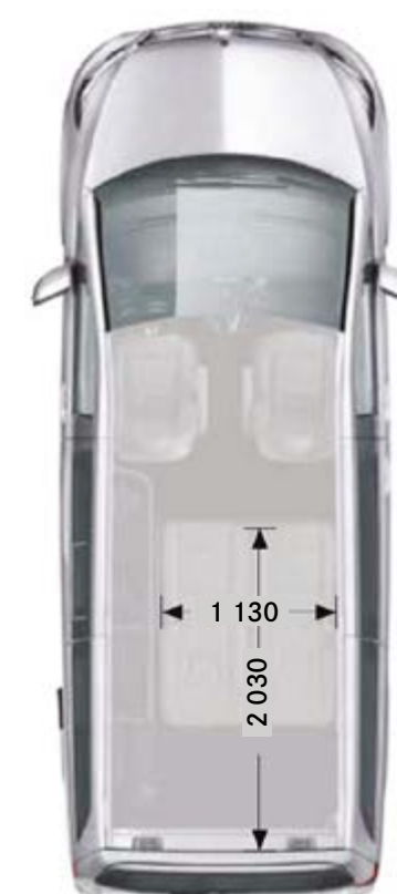
Banquette en position couchette
