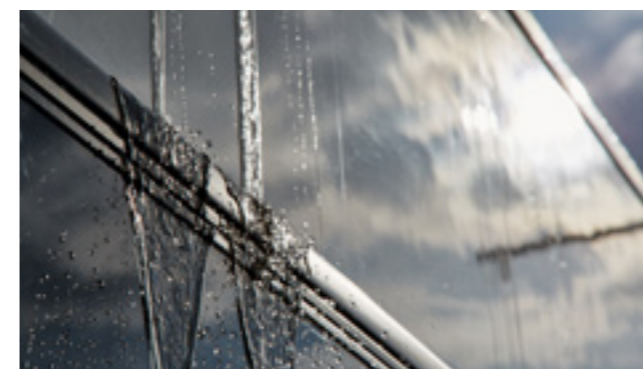
Test d'étanchéité contre l'infiltration d'eau à 100 % des camping-cars sortant de production, avant livraison.
