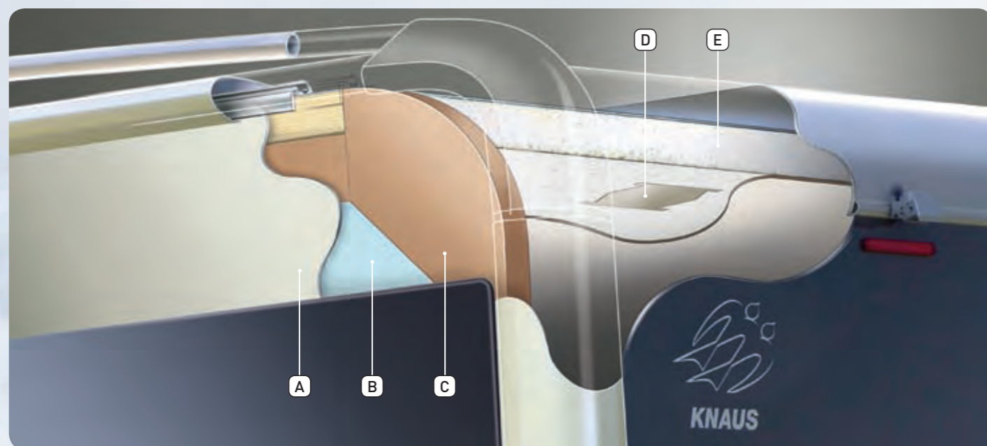
● Sans son enveloppe: cette représentation montre la géniale structure en sandwich de cloisons extérieures
