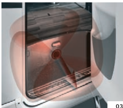
Porte d'entrée : Sortie d'air chaud pulsé dans le marchepied de la porte d'entrée
