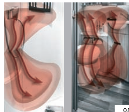
Cabinet de toilette et douche : Air pulsé chaud et bac à douche chauffé
