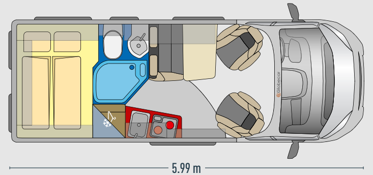
Grande dînette | Idéale pour accueillir 4 personnes
