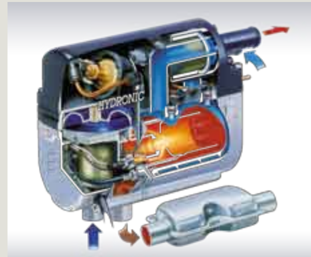
Riscaldamento FRANKIA Polar ad acqua Eberspächer
