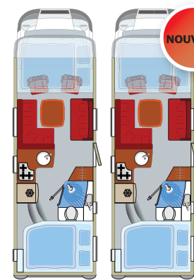
Terrestra A 720 HB Longueur 7,39 m
