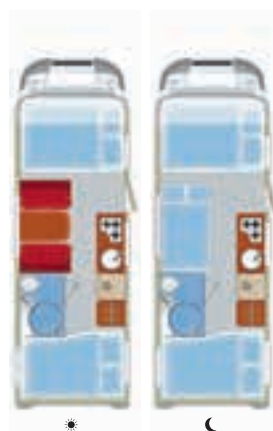
Terrestra A 690 HB Longueur 7,06 m
