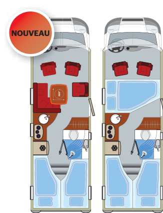
Contura Style CS 710 EB Longueur 7,39 m
