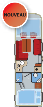
Integra 810 HB Longueur 8,44 m
