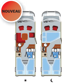
Terrestra T 710 EB Longueur 7,33 m
