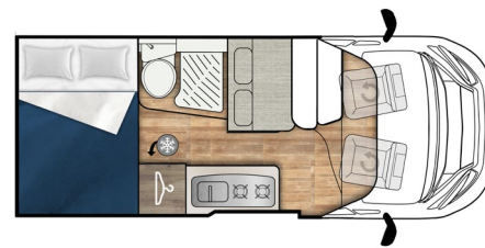
E-Van 2 ↔ 5990 mm
