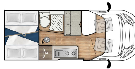
E-Van 5 Premium/Trend ↔ 5990 mm
