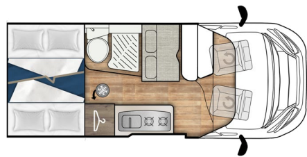
E-Van 5 ↔ 5990 mm
