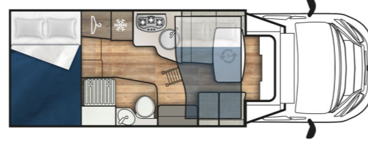
T-loft 530 ← 7450 mm I 2350 mm
