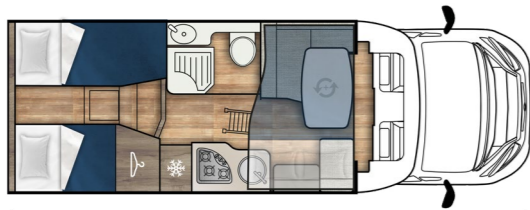
Baron 565 ← 6990 mm I 2350 mm
