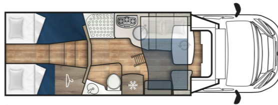
T-loft 530 ← 7450 mm I 2350 mm
