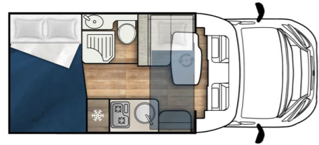
Baron 565 ← 6990 mm I 2350 mm
