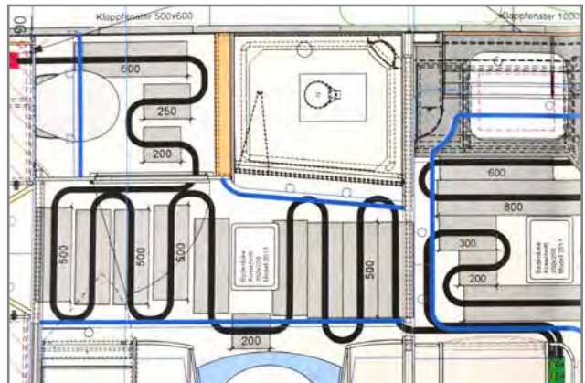
CHAUFFAGE PAR LE SOL DEUX ZONES
