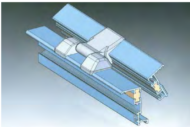
PROFILÉS SANS PONTS THERMIQUES
