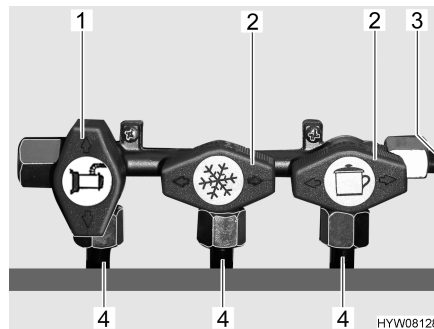
Fig. 52 Position des robinets d'arrêt de gaz (exemple)
