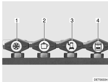
Fig. 51 Symboles des robinets d'arrêt de gaz
