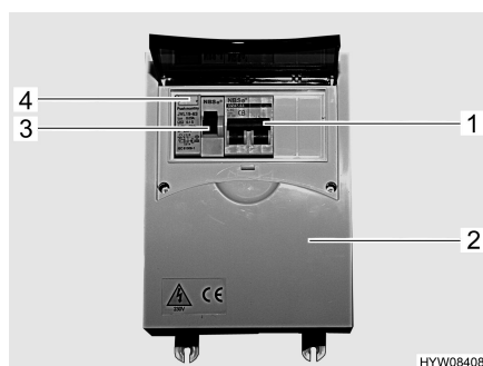
Fig. 55 Coffret de fusibles 230 V avec disjoncteur de protection de circuit et disjoncteur FI
