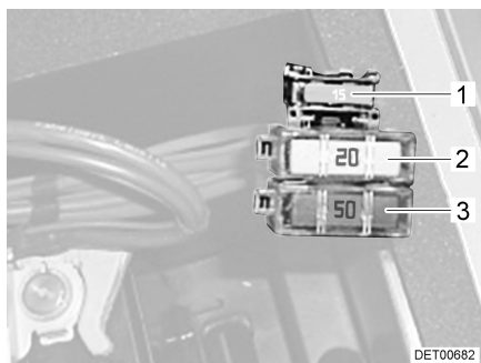
Fig. 58 Fusibles de la batterie de démarrage
