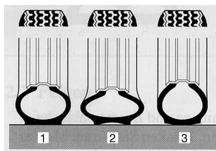
Fig. 112 Surface de contact du pneu
