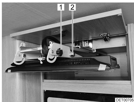
Fig. 29 Écran plat dans niche pour téléviseur
