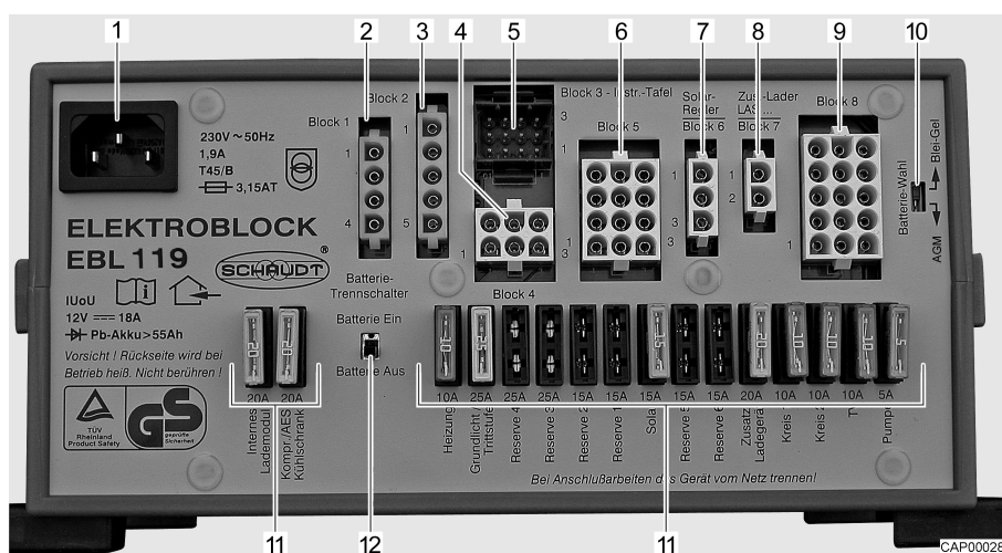
Fig. 53 Bloc électrique (EBL 119)
