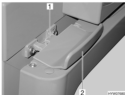
Fig. 77 Dispositif de verrouillage de la porte du réfrigérateur, fermé (Thetford)
