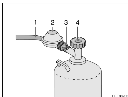
Fig. 50 Raccord bouteille de gaz
