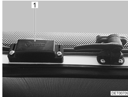
Fig. 63 Interrupteur de sécurité
