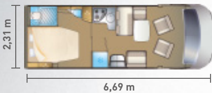
I650LC - 4 pl. - 3,5 T.
