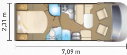
I690LC - 4 pl. - 3,5 T.
